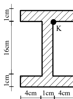
Przekroj nr 4
