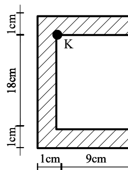
Przekroj nr 8
