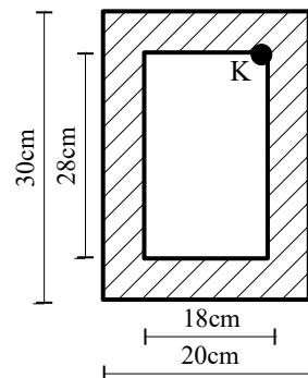
Przekroj nr 8
