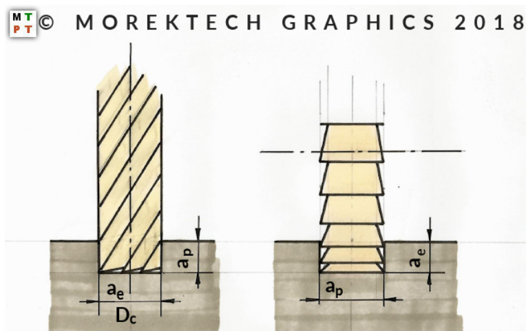
Ilustracja 3. Po lewej stronie frezowanie czołowe, a po prawej obwodowe – interpretacja szerokości i głębokości frezowania.
