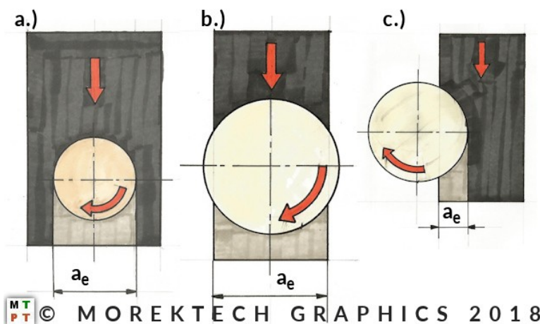
Ilustracja 4. Frezowanie czołowe: a.) pełne, b.) niepełne symetryczne i c.) niepełne niesymetryczne.
