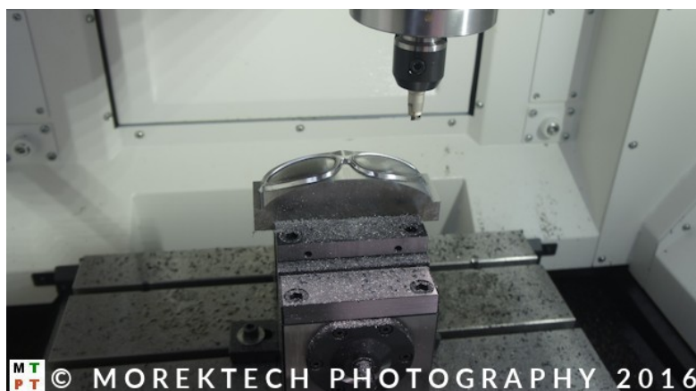
Ilustracja 6. Przykład obróbki powierzchni o bardziej skomplikowanym kształcie. Frezarskie centrum CNC firmy MAZAK.
