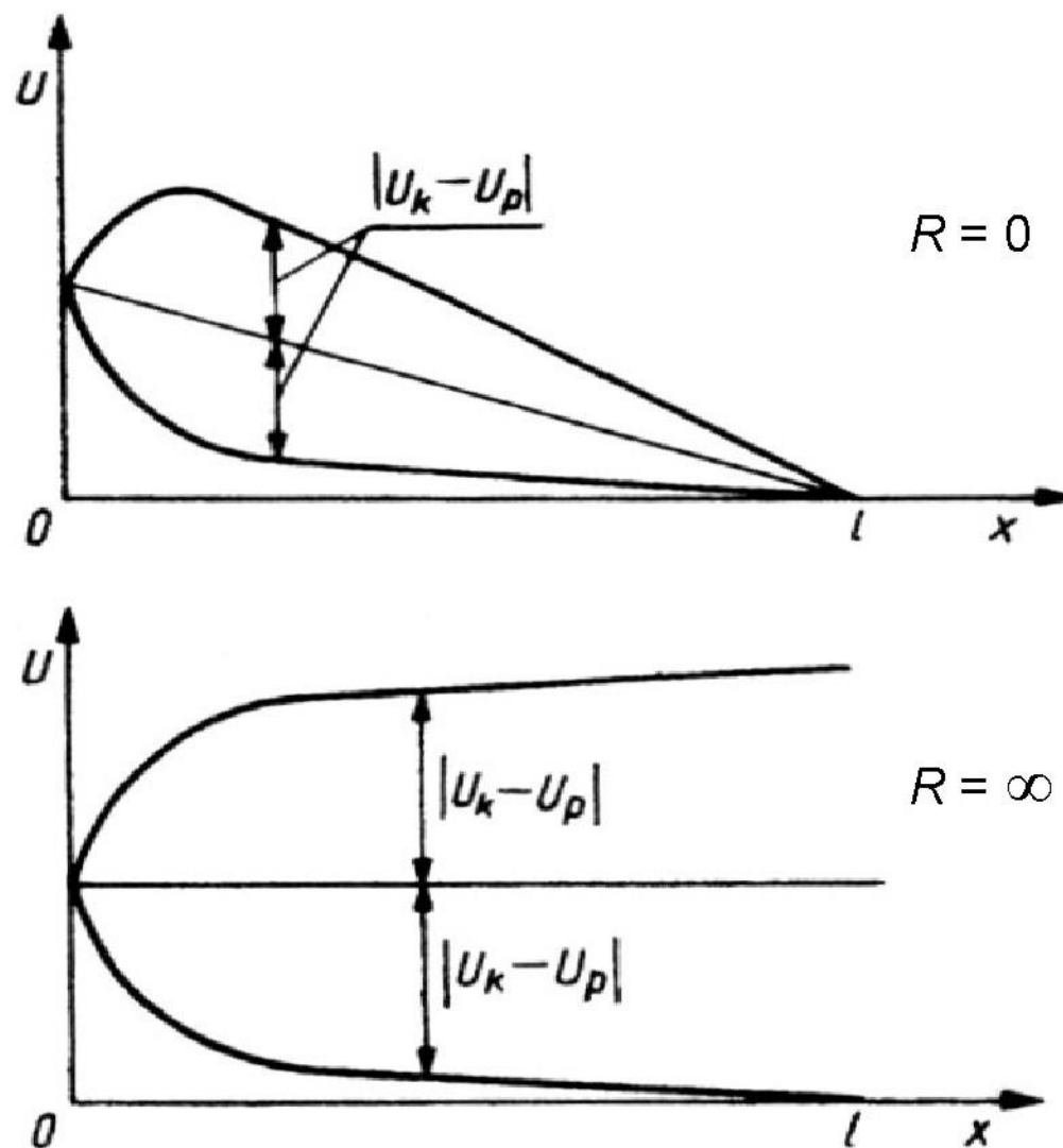
Rozkład przejściowy fali przepięciowej w uzwojeniu transformatora, obwiednie drgań
