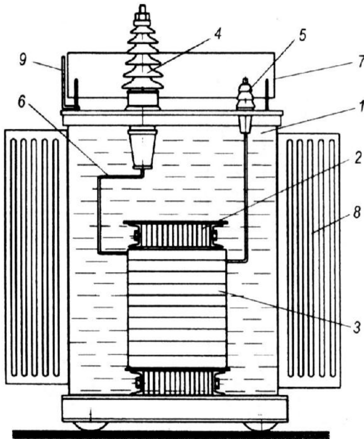
Szkic transformatora olejowego napowietrznego SN/nn: 1 - olej w kadzi, 2 - rdzeń, 3 - uzwojenia, 4, 5 - izolatory przepustowe, 6 - wyprowadzenie początku uzwojenia, 7 - konserwator oleju, 8 - radiatory, 9 - wskaźnik oleju.
