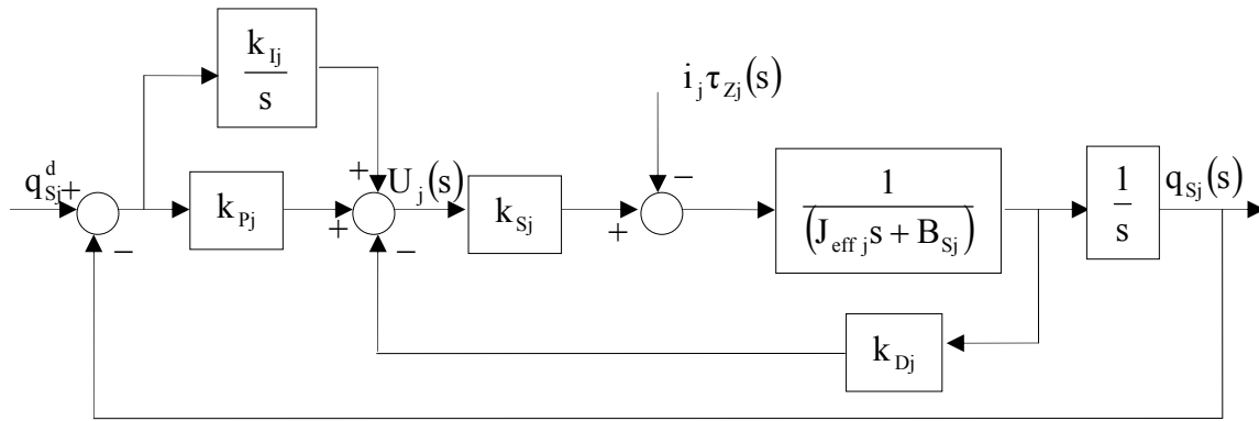
Rys.3. Schemat blokowy układu zamkniętego ze sterowaniem PID
