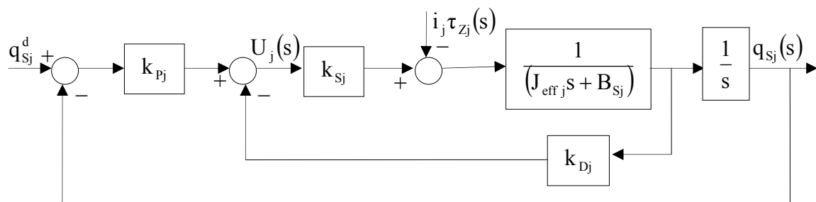
Rys.2. Schemat blokowy układu zamkniętego ze sterowaniem PD
