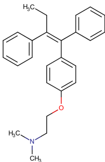
Rysunek 3. Tamoksyfen – wzór strukturalny, struktura 3D oraz podstawowe identyfikatory chemiczne.
