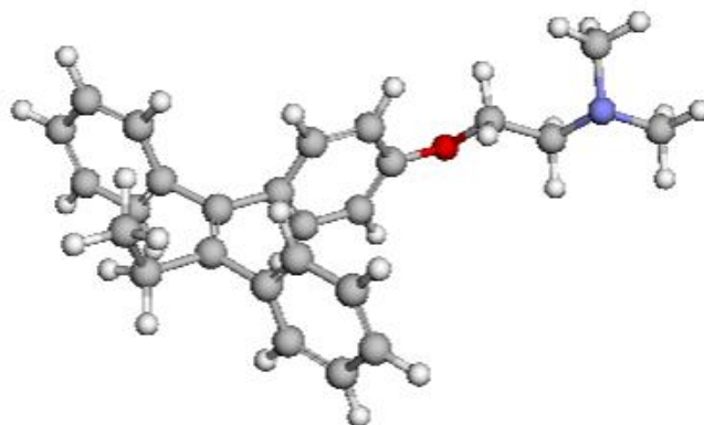
Rysunek 3. Tamoksyfen – wzór strukturalny, struktura 3D oraz podstawowe identyfikatory chemiczne.
