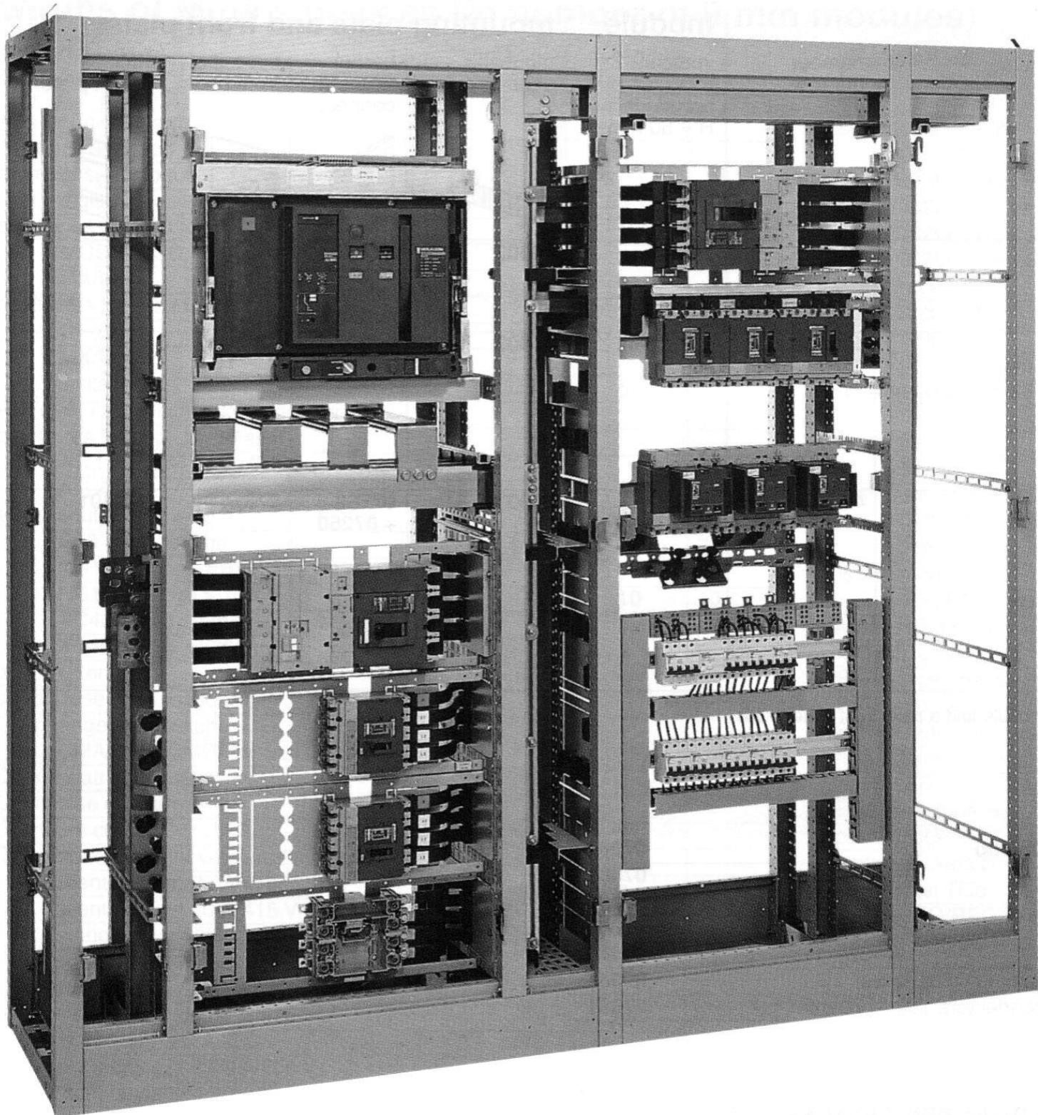
Widok rozdzielnic po zdjęciu osłon.
