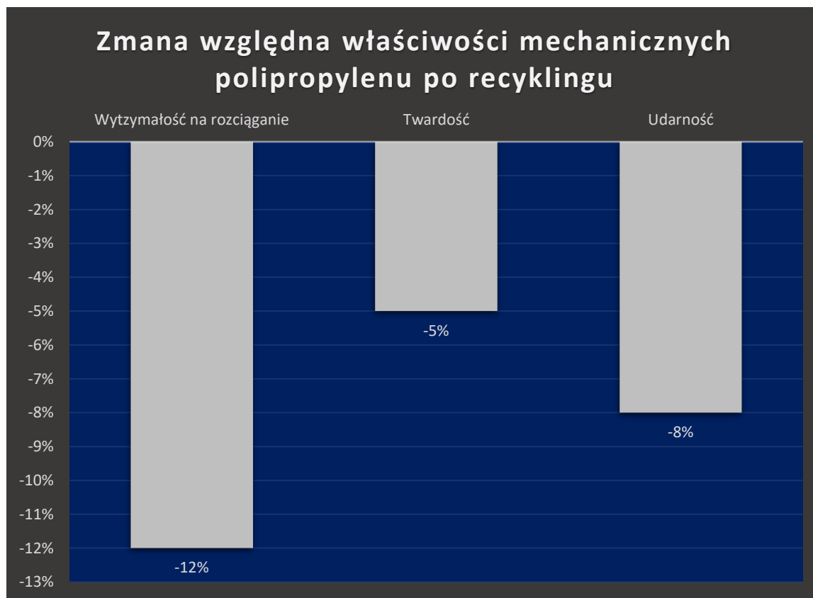
Wykres 1. Wykres zmiany względnej właściwości mechanicznych
